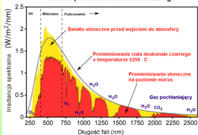
Widmo promieniowania słonecznego
